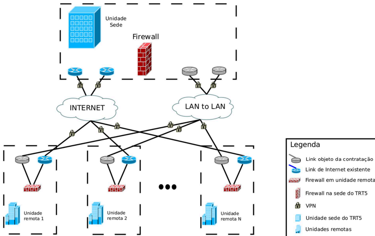
Figura 1. Topologia da solução de redundância composta por links de Internet da ITS e links dedicados Ponto-a-Ponto objeto da contratação.
