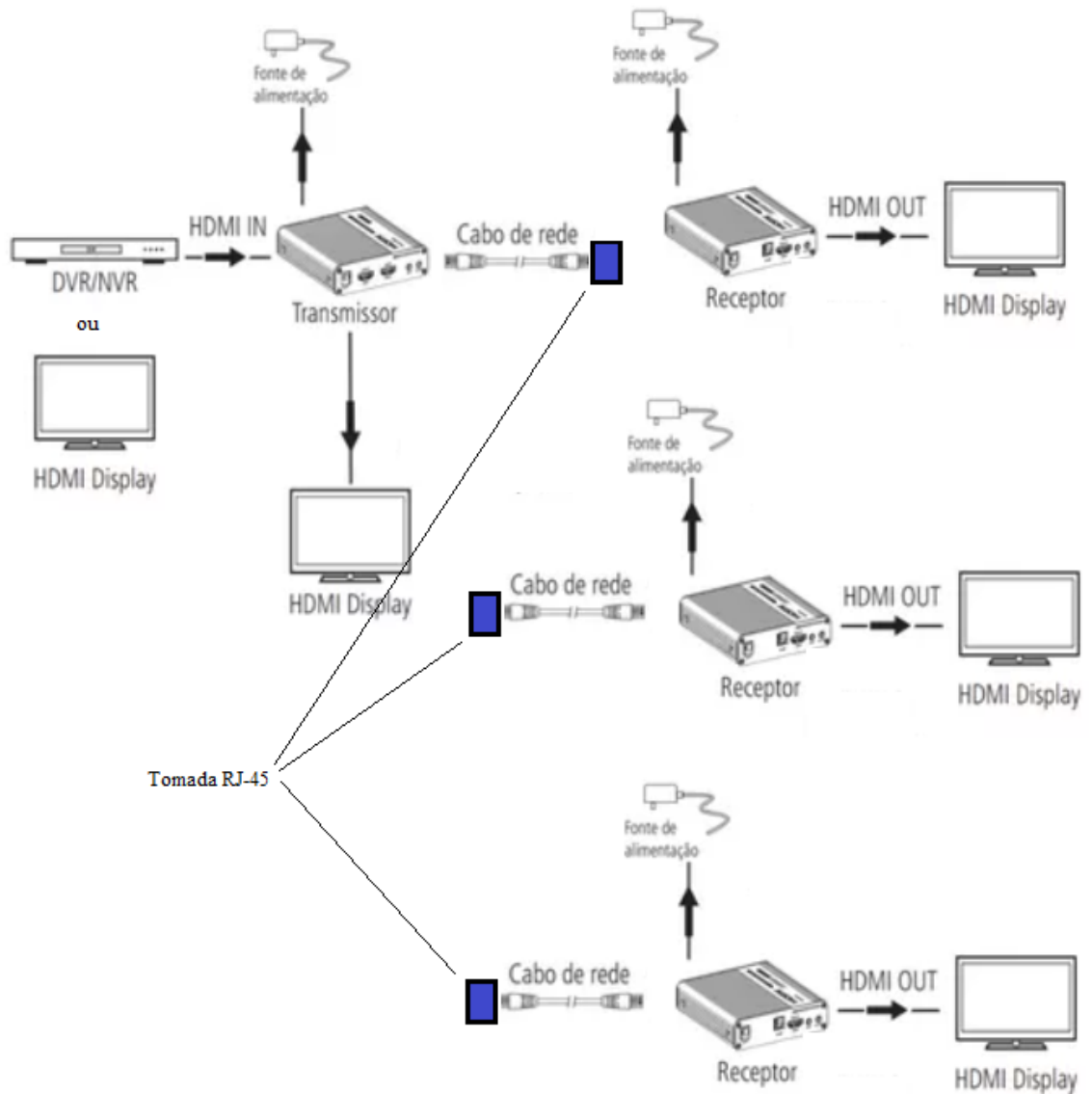
Figura 2 - Arquitetura da Solução HDMI IP VEX 3120 da Intelbrás via Rede Lógica
